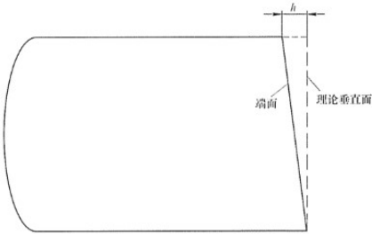
图 2 圆铸锭端面切斜度测量示意图
